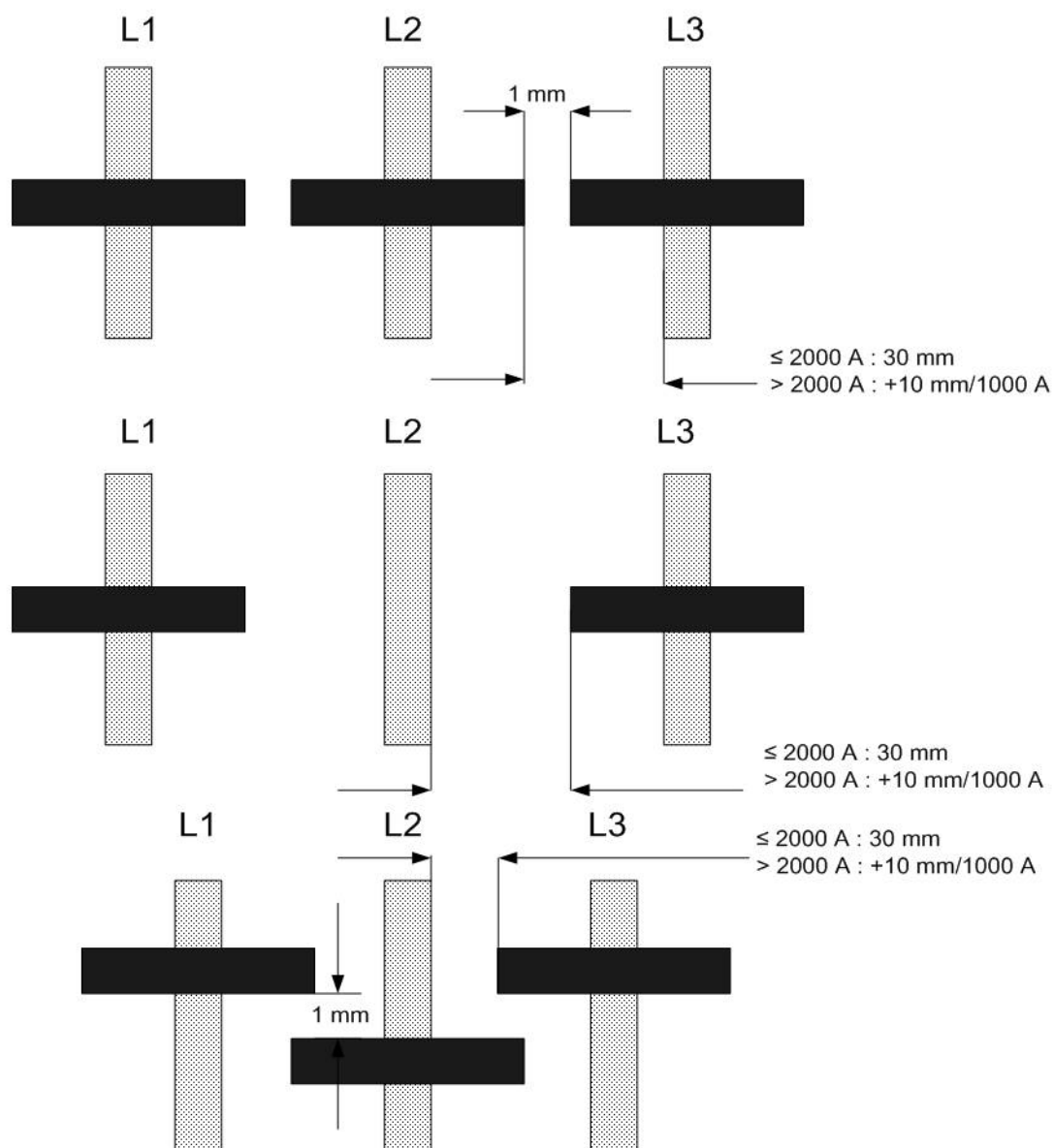
Figur 5 Krav til strømtransformatorers avstand
